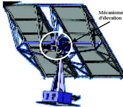
Fig. 4: Structure porteuse - vue arrière et emplacement du vérin
