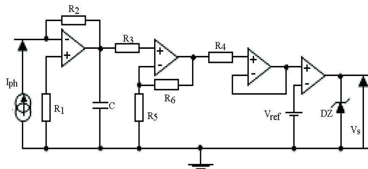
Fig. 10: Circuit de conditionnement
