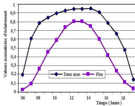
Fig. 15: Eclairement en fonction du temps (14/06/07)
