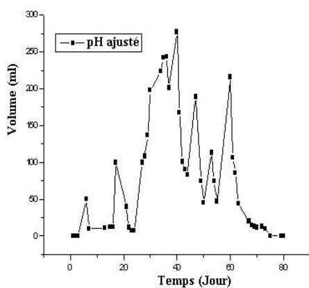
Fig. 4a: Evolution du volume de biogaz en fonction du temps
