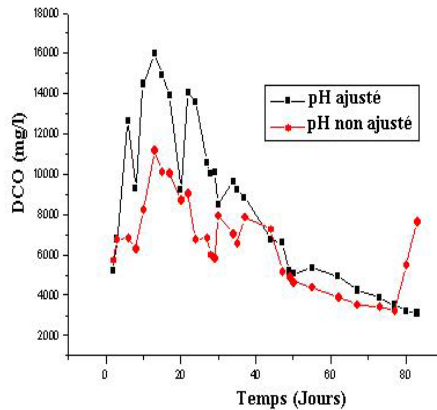
Fig. 5: Variation de la DCO en fonction du temps
