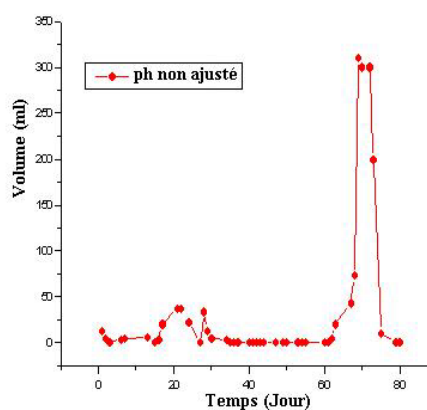
Fig. 4b: Evolution du volume de biogaz en fonction du temps
