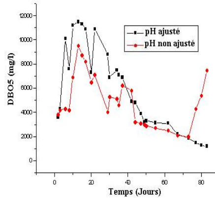
Fig. 6: Variation de la DBO 5 en fonction du temps
